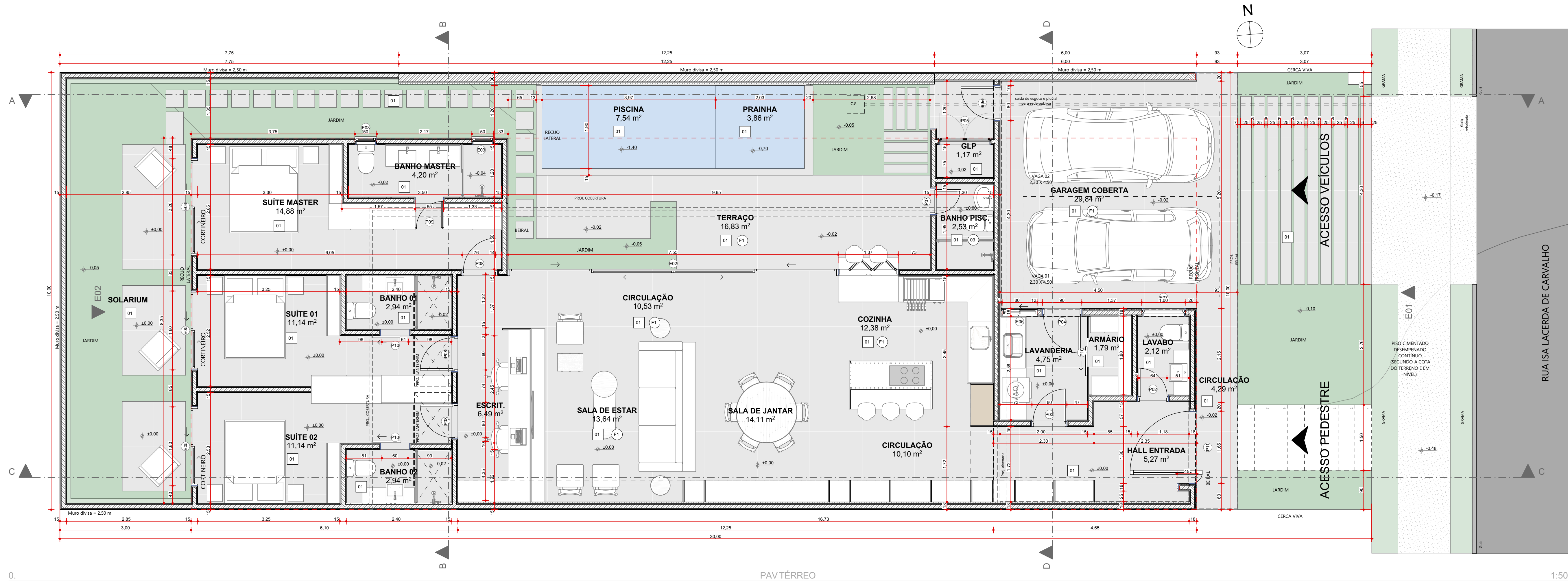
0. PAV. TÉRREO 1:50
