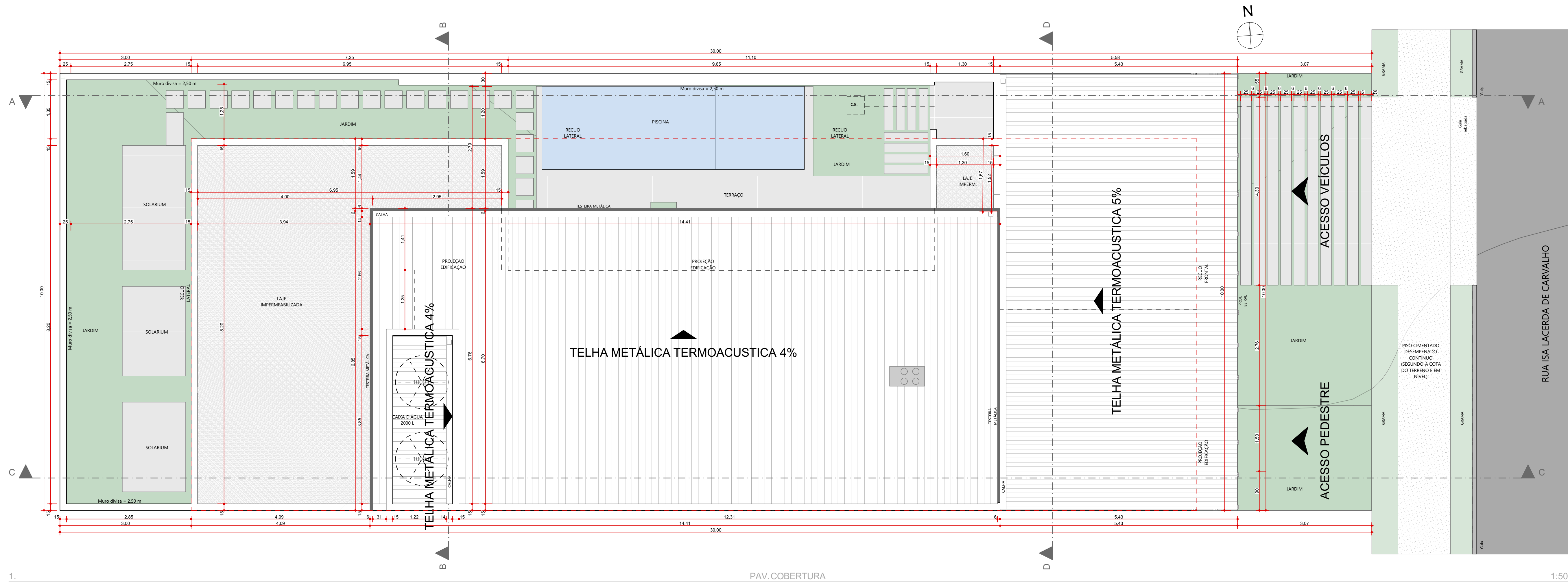
1. PAV. COBERTURA 1:50
